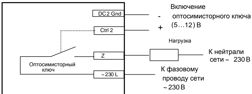
(б) исполнения Ctrl2_230_L и Ctrl2_230_H
