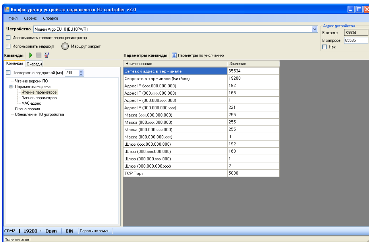
Рис. 1.5. Параметры Ethernet адаптера
