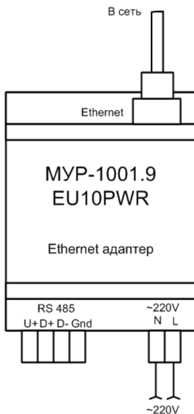
Рис. 1.1. Подключение Ethernet-адаптера к сети
