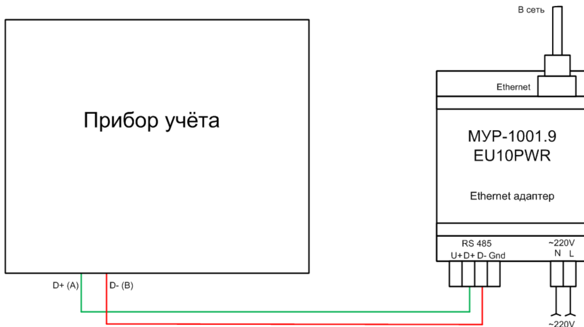
Рис. 2.1. Подключение прибора учёта к Ethernet-адаптеру
