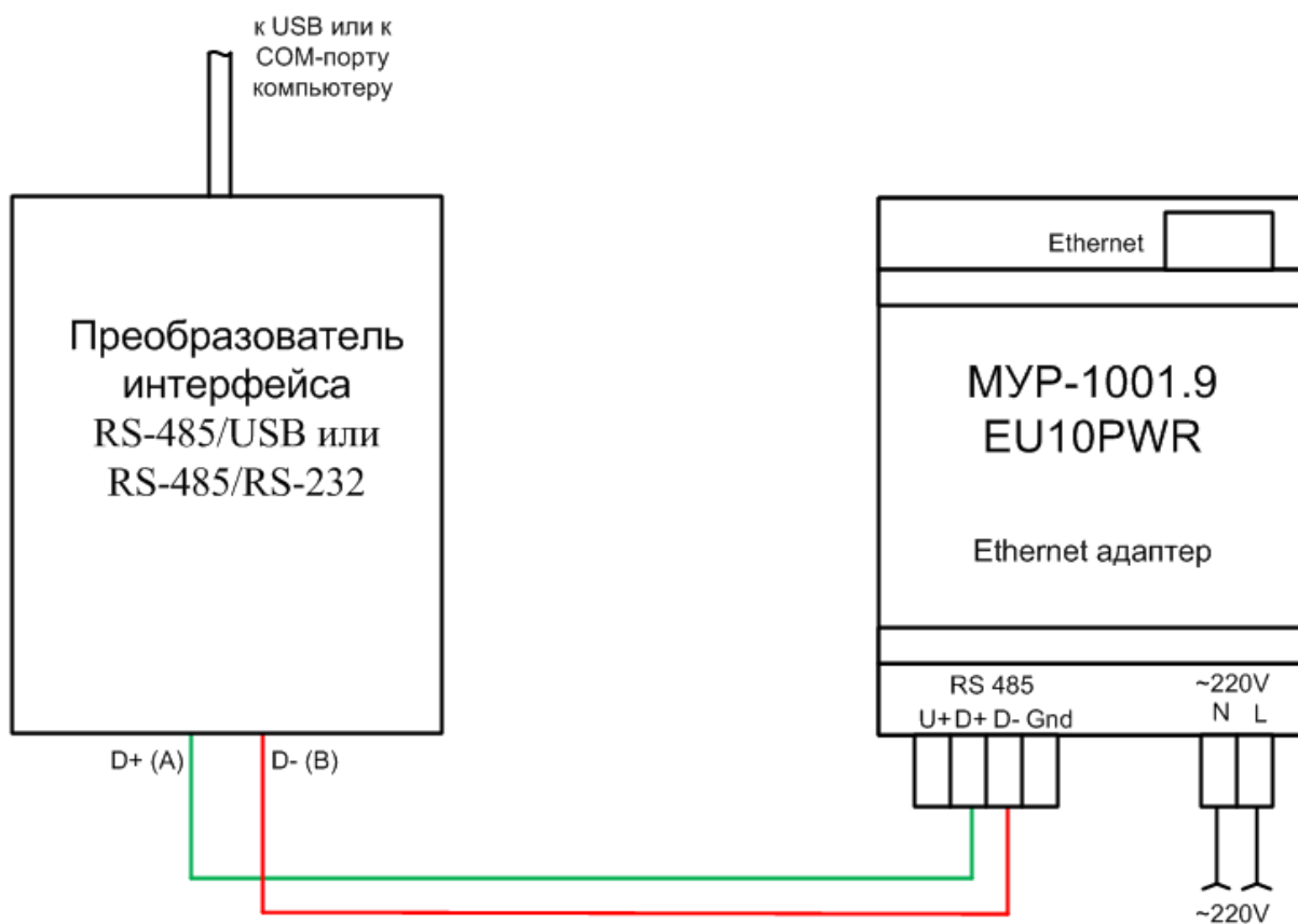
Рис. 1.3. Подключение Ethernet-адаптера к компьютеру
