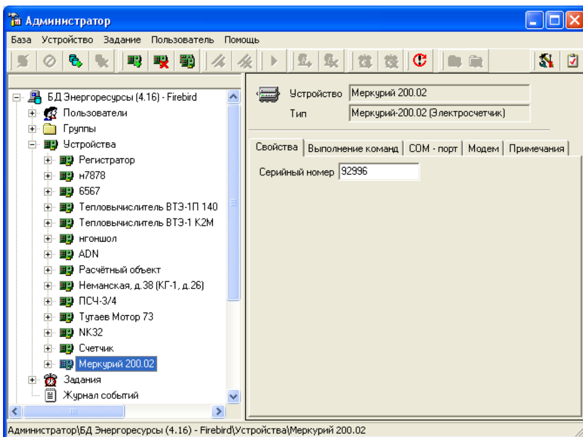
Рис. 4.3. Вкладка Свойства.
