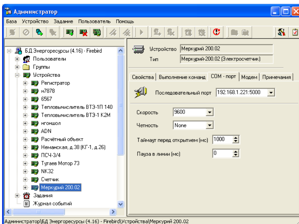
Рис. 4.4. Вкладка COM-порт.
