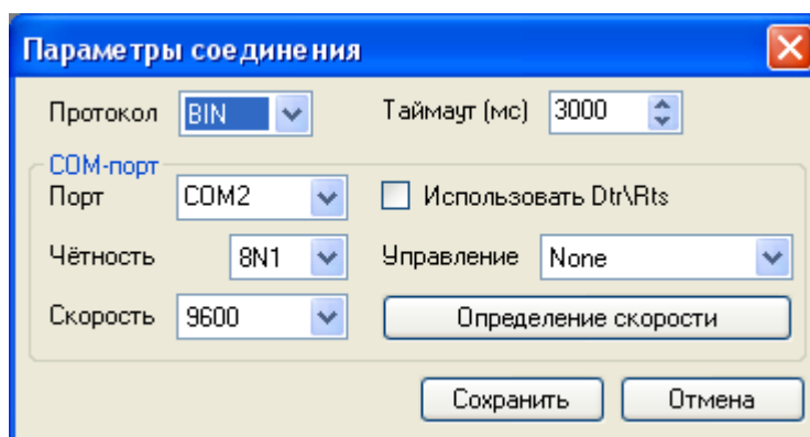
Рис. 1.4. Параметры соединения
