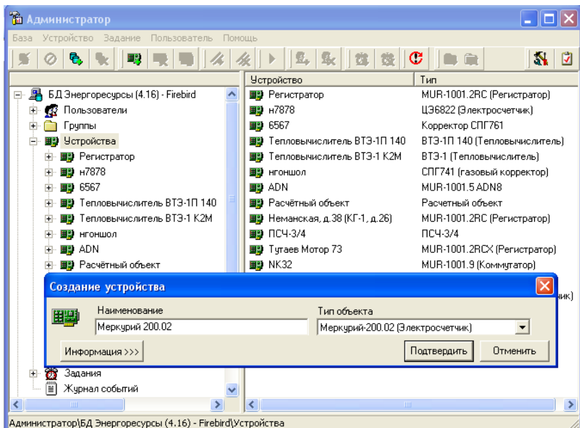
Рис. 4.2. Создание устройства.
