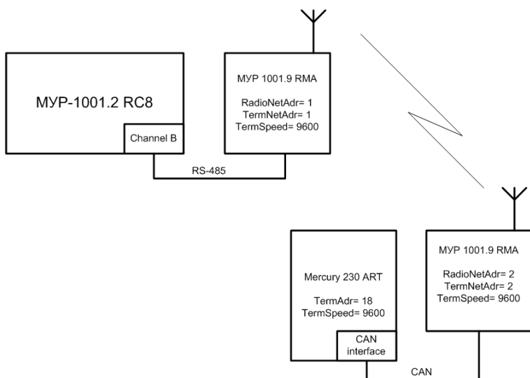
Рис. 3.1 Схема АСКУЭ
