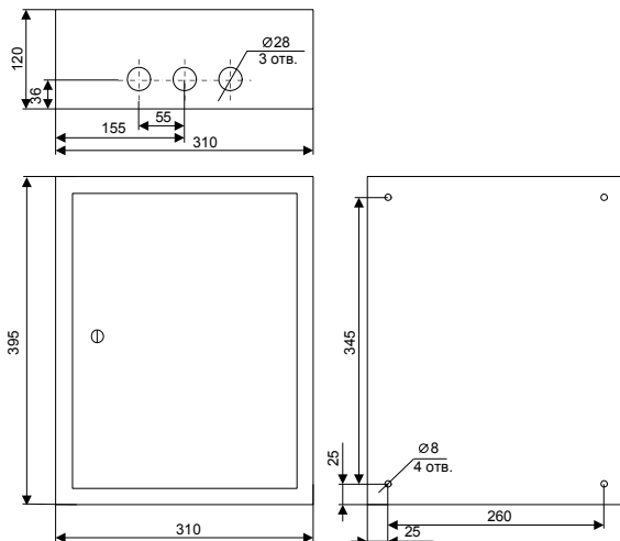
Рис.1 Установочные размеры
